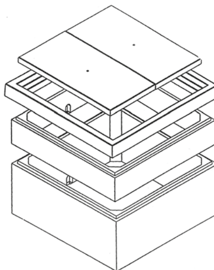
Variante trappon tôle 125 KN
