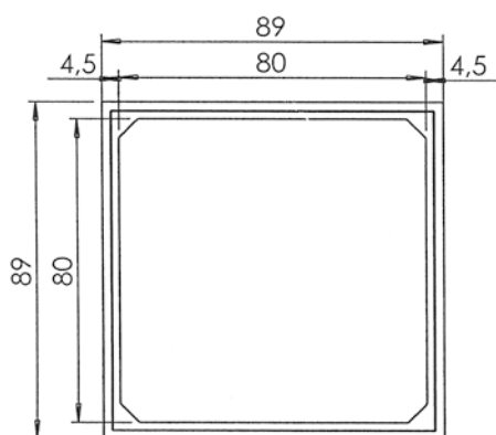
Variante trappon tôle renforcée 250 KN
