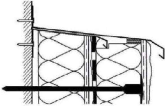
Figure 2 : Exemples de traitement des points singuliers en surisolation
