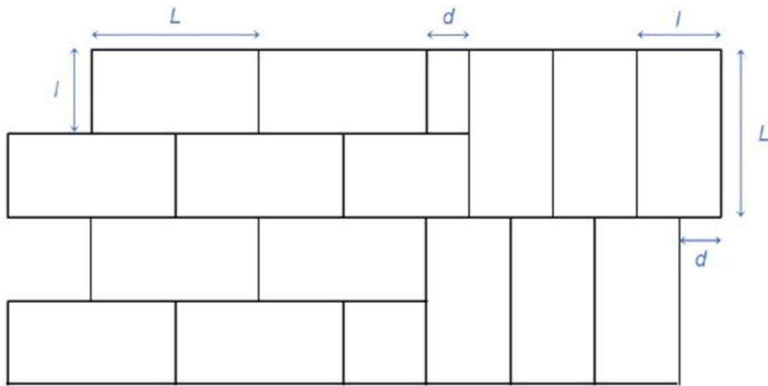
Figure 3 : Juxtaposition des poses verticale et horizontale des panneaux isolants sur une même façade
